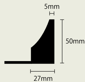
【フレーム断面図】
